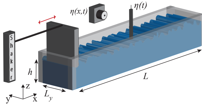
Figure 1. Dispositif expérimental : forçage par batteur, et mesure du champ d'ondes par une sonde localisée, \eta(t) , et par une caméra latérale visualisant l'interface \eta(x, t) [2]. Cambrure typique des vagues \epsilon \sim 0.05 .
